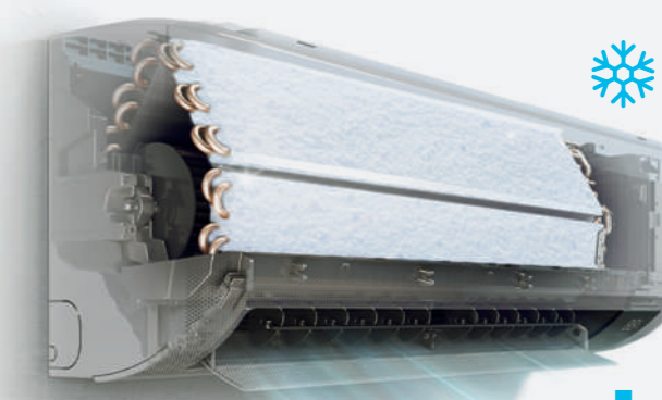
Namrznutý Výmenník Tepla (-15°C)
